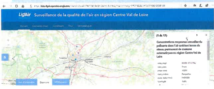
Concentrations moyennes annuelles de polluants dans l'air ambiant issues du réseau permanent de mesures automatiques en région Centre-Val de Loire
