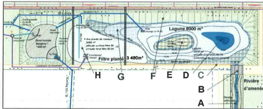
N.B. : Sur le plan du fonctionnement hydraulique, le projet reste identique (§ 2.3). Les lettres A à H pointent les éléments clés de la conception (développés en partie 3).
